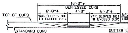
ELEVATION
